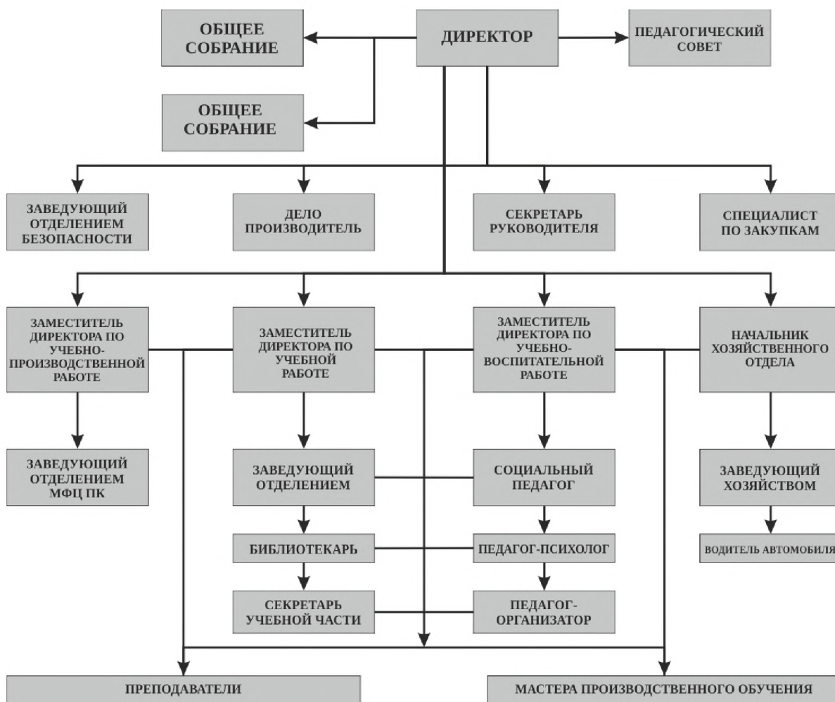
Рис.1 Структура управления
